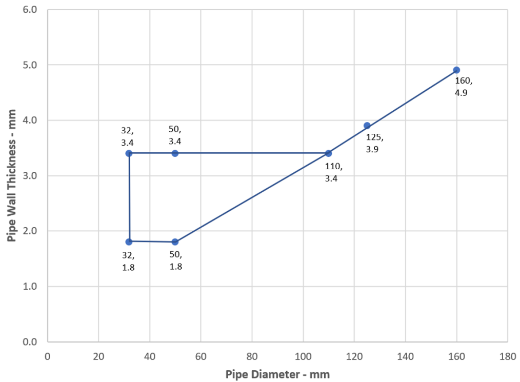
Geberit Silent PP Pipes – U/C
