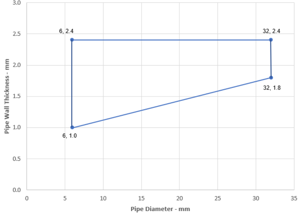
PVC-U Pipes - EI 60 U/C
